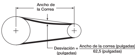
Figura 7 — Tensión de la Correa
