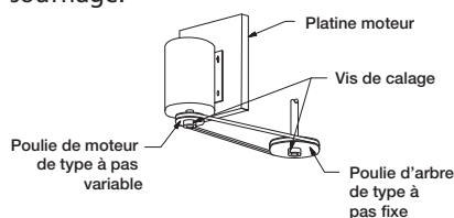
Figure 5 — Schéma de l'entraînement
