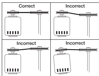
Figure 6 — Alignement des poulies
