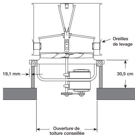
Figure 3 — Pose en toiture typique
