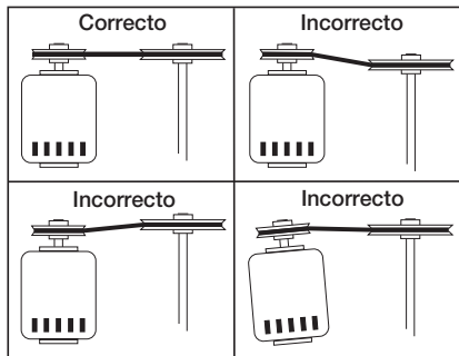
Figura 6 — Alineación de las Poleas
