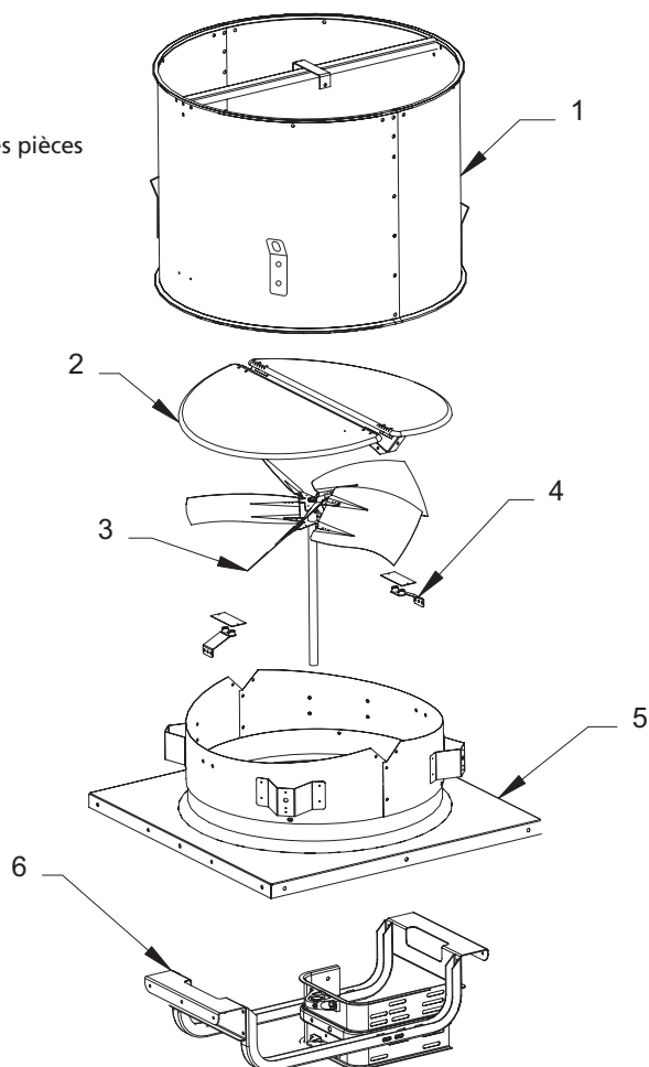
Figure 8 — Pièces de rechange pour tourelles d'extraction axiales à courroie et rejet vertical
