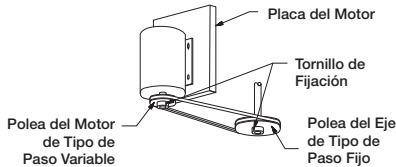
Figura 5 — Diagrama del Paquete de Accionamiento
