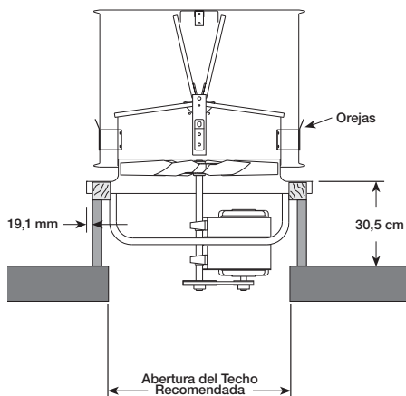
Figura 3 — Montaje en Techo Típico
