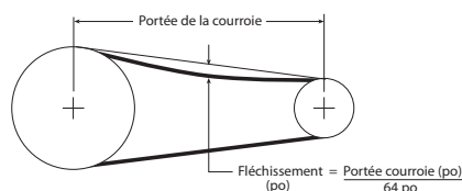
Figure 7 — Tension de la courroie
