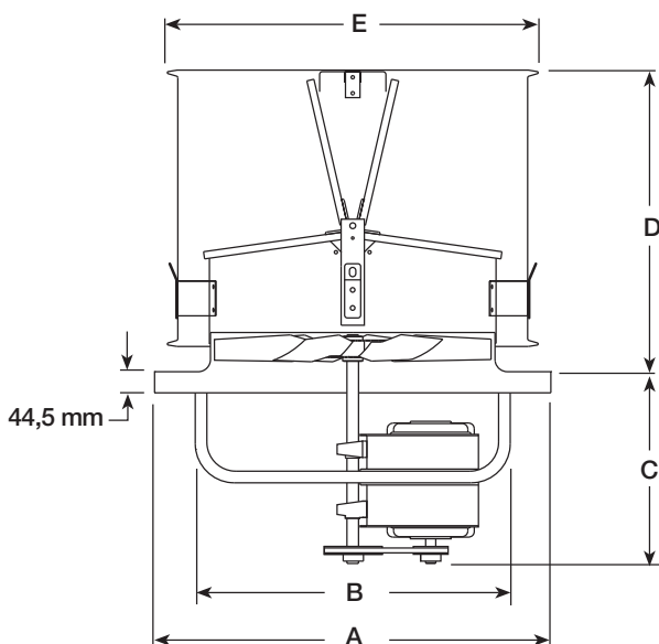
Figura 1 — Dimensiones
