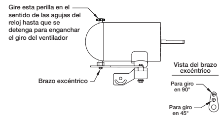
Figura 8 — Modo de Giratorios
