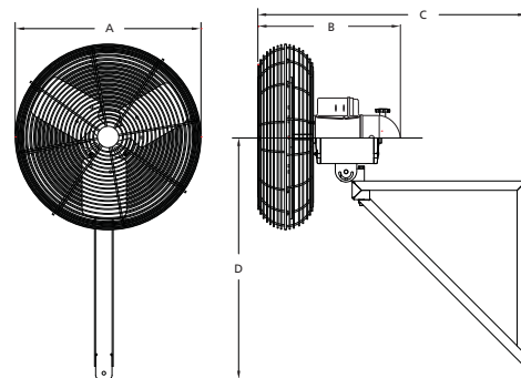
Figure 3 — Dimensions du 3PEG9 et du 3PEH1
