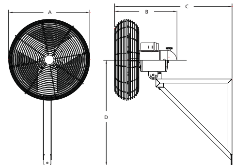
Figura 3 — Dimensiones de 3PEG9 y 3PEH1
