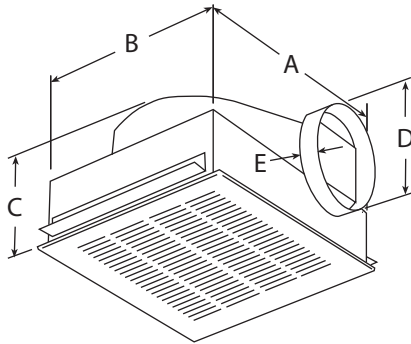
Figura 1 — Dimensiones
