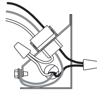
Figura 5 — Cableado Correcto
